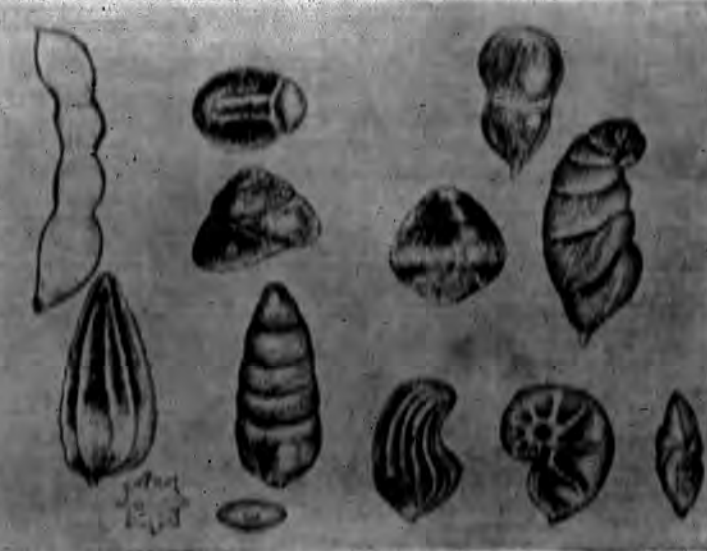
نقشه بعضی از فرامیهای فرها که به اندازه های بسیار کوچک در طبقات مختلف زمین وجود دارند
